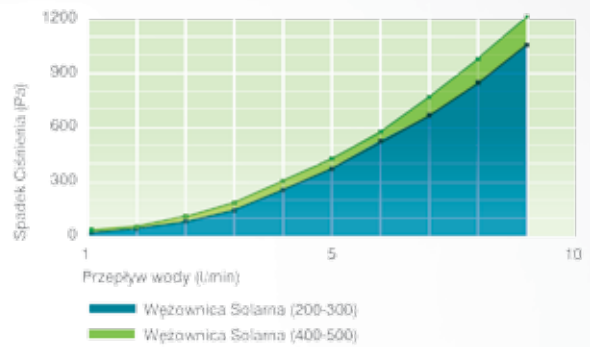
Wężownica Solarna – Wykres Spadku Ciśnienia
