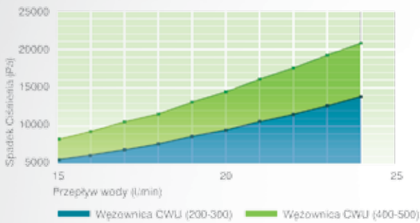
Wężownica CWU – Wykres Spadku Ciśnienia
